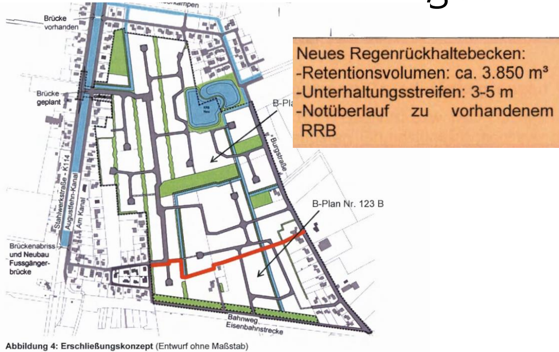
Abbildung 4: Erschließungskonzept (Entwurf ohne Maßstab)
